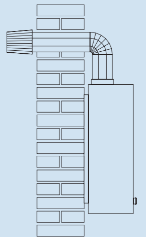
Gesloten geiser: rookgasafvoer en luchttoevoer via buitenmuur of dak
